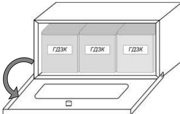
Рисунок 1 Контейнер для самоспасателей ГДЗК-03, внешний вид в закрытом и открытом состоянии.
