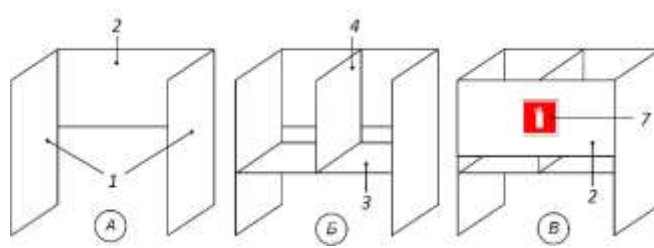
Рис. 3 Сборка П-10/2, П-15/2, П-20/2
