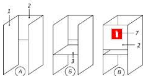
Рис. 2 Сборка П-10, П-15, П-20
