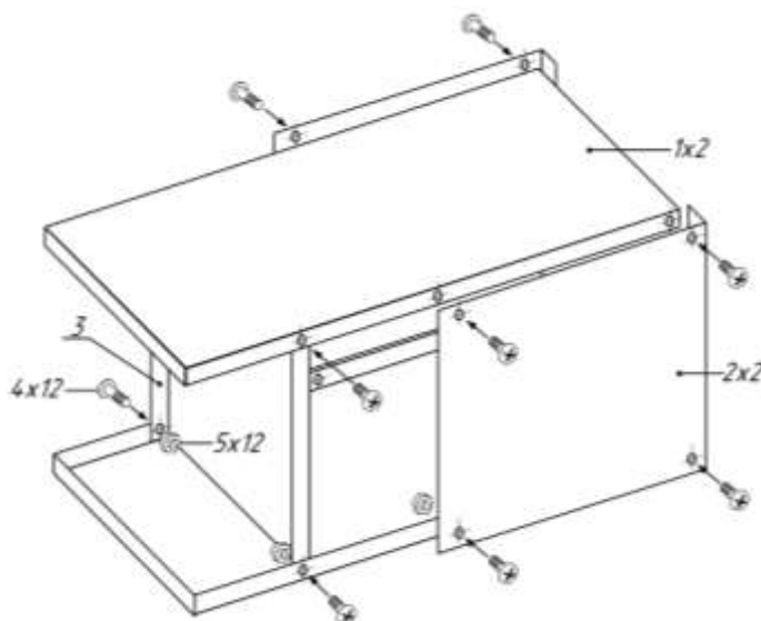
Рис. 1 Подставка под огнетушитель сборно-разборная
